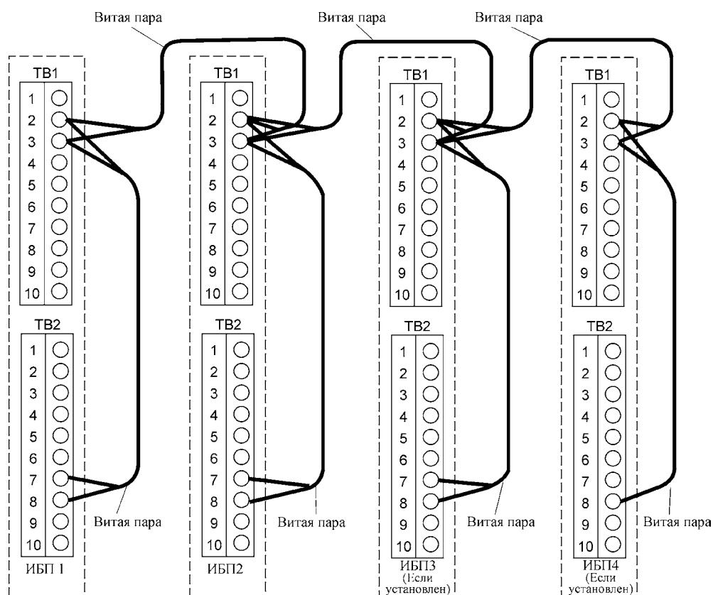
Рис. 43. Сигнальные кабели синхронизации ИБП для работы в режиме байпаса.
