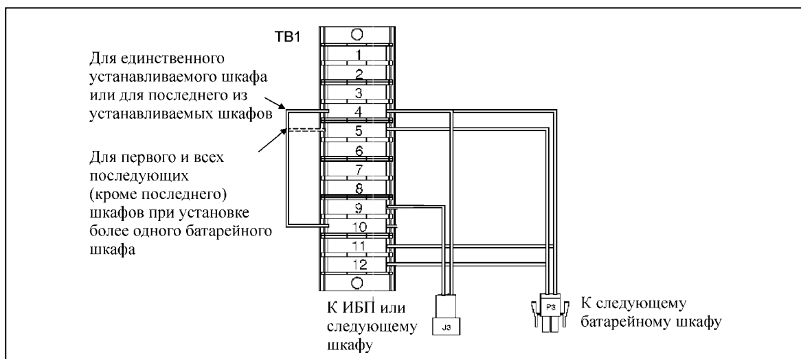
Рис. 17. Схема подключения сигнальных кабелей к колодке TB1.
